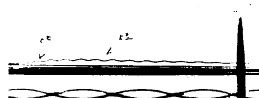
Fig. 17. No. 165. \text{H}_2:\text{O}_2=1:8 , P=15\text{ cmHg}
