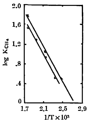
Hg(CH 3 ) 2 + (ネオペンタン) C 2 H 6 に於ける CH 4 生成 o: エタン; x: ネオペンタン
