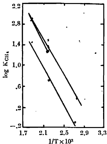
Hg(CH 3 ) 2 + D 2 に於ける CH 4 生成 x: 通常の光の強さ; o: 弱い光の強さ △: 充填容器
