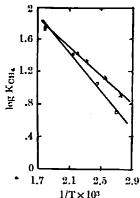
Hg(CH 3 ) 2 + ブタン(o); イソブタン(x) に於ける CH 4 生成
