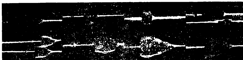
第九圖 左上より右下へ順次に、 H_2 (第一表實驗2); ヘプタン(20); メタン(4); エチレン(上方が實驗8); ベンゼン(10及11); ヘクサン(15); チクロヘキサン(17); チクロヘキセン(18)。
