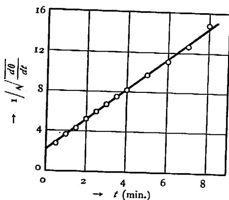
Fig. 3.—Expt. 4.
