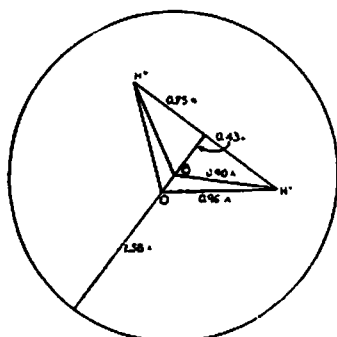
第四圖 水分子模型
