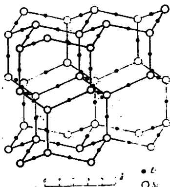
第三圖 Tridymite 格子
