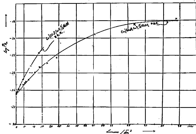
第十一図 \text{Cu}|\text{Cu}_2\text{O}, \text{Cu}_2\text{S} 電池の \log P_H と照度との関係
