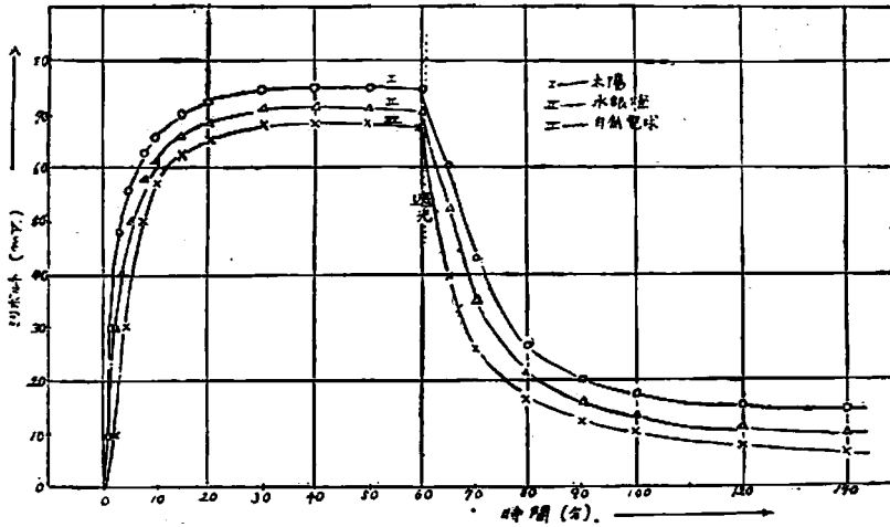
第二圖 光源の種類と \text{Cu}/\text{Cu}_2\text{O} 溶液の Becquerel 効果
