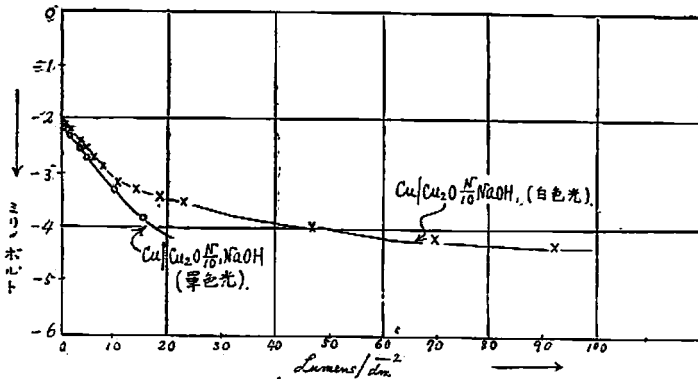
第八圖 光の強さと \text{Cu}|\text{Cu}_2\text{O} \frac{\text{H}}{10} \text{NaOH} 電極との関係
