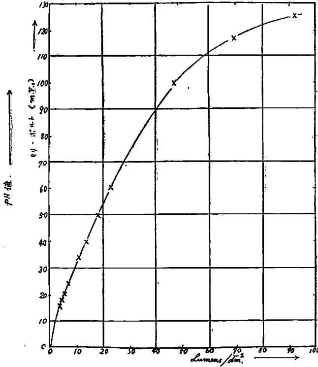
第三圖 光の強度と \text{Cu}|\text{Cu}_2\text{O}, \text{CuO} \frac{\text{N}}{10} \text{NaOH} 電極の光効果 との関係
