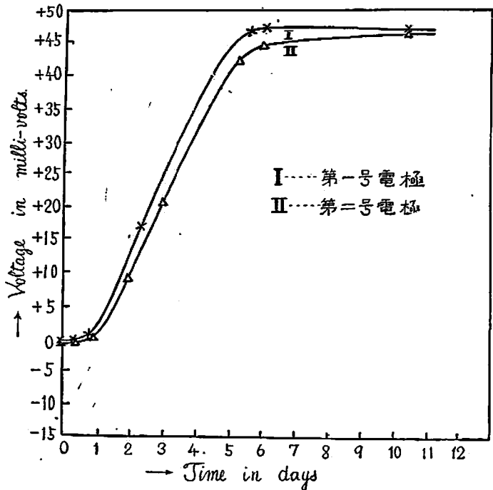
第 六 圖 (酸化銅電極の單極電位の 變化に伴ふ光効果の變化)
